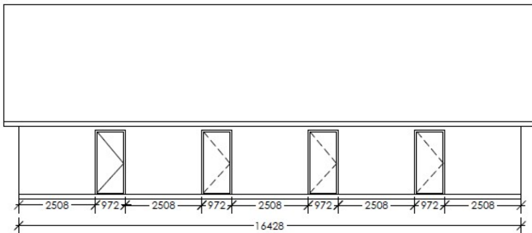
Facade mod Syd, mod ejers bolig.
